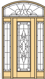
I 68-1/2 x 124 6623-131 R=66-3/8
