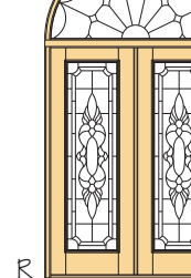
R 74-1/4 x 137-3/4 7236-309B R=37-1/8
